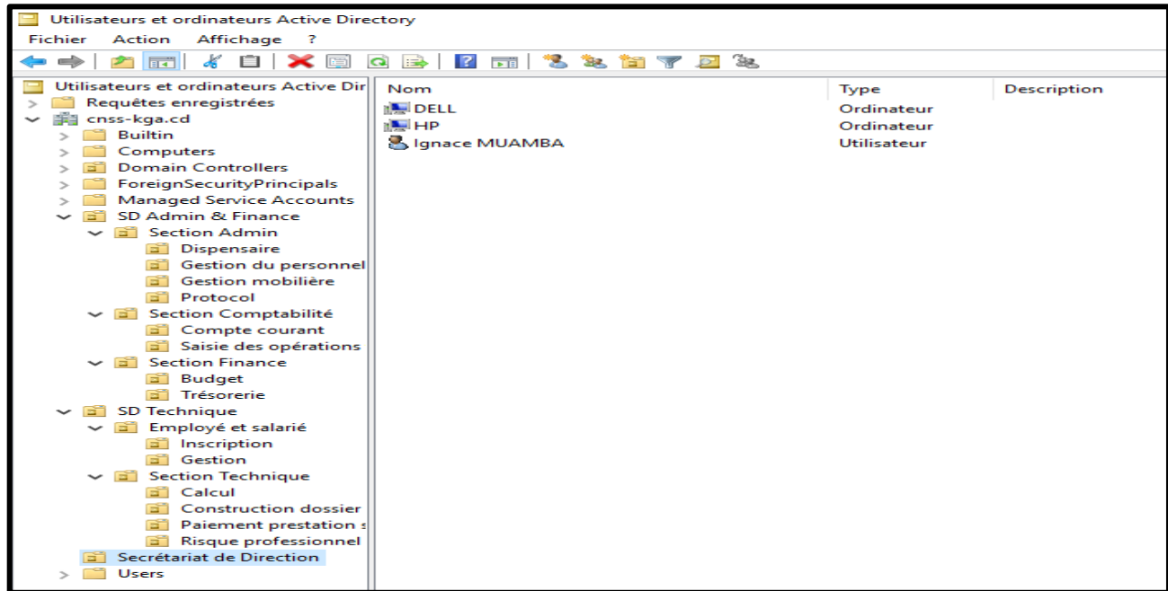
Figure 18 : Unités d'organisation.
