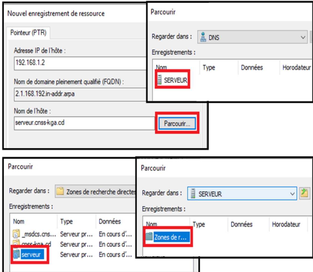
Figure 13 : Processus de création d'un alias.
