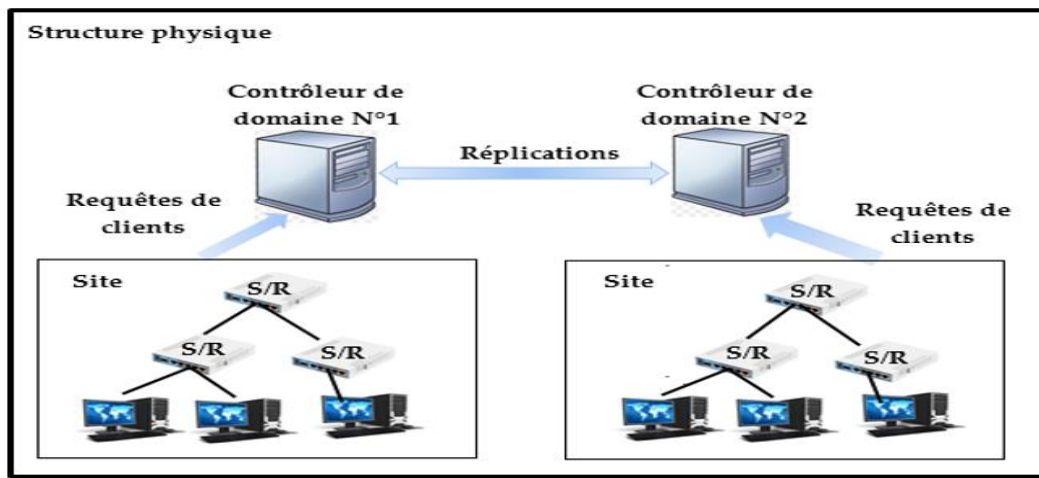
Figure 1 : Structure physique d'un Active Directory.
